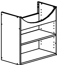
ALLASKAAPPI 568 x 300
