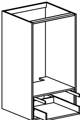
ASTIANPESUKONEKOMERO 1120x570
