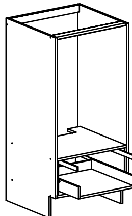
ASTIANPESUKONEKOMERO 1270x570
